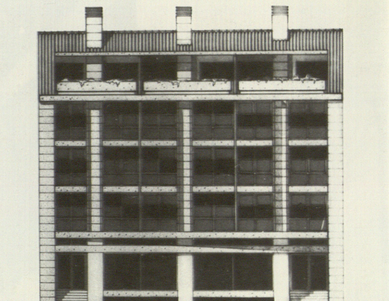
ALZADO (CALLE HERRADURAS)
